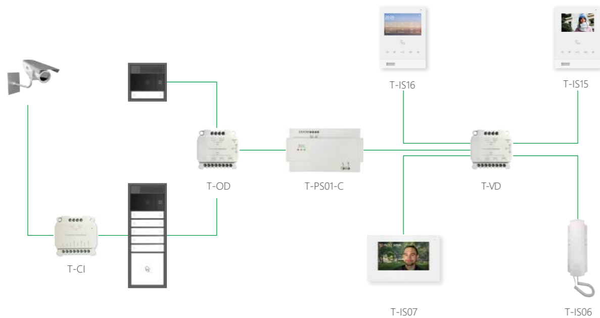
"Звезда"
