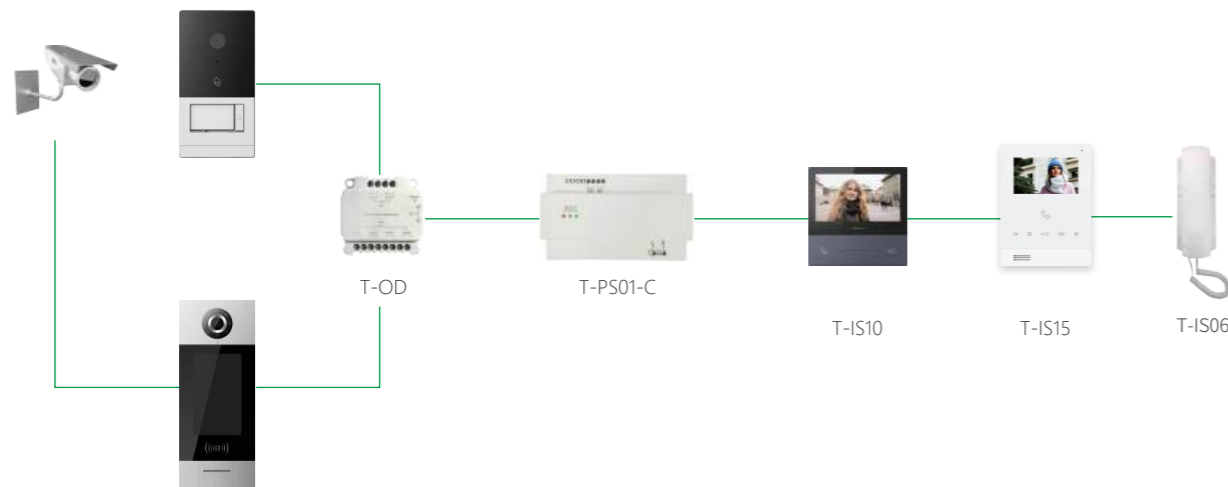
Последовательное соединение
